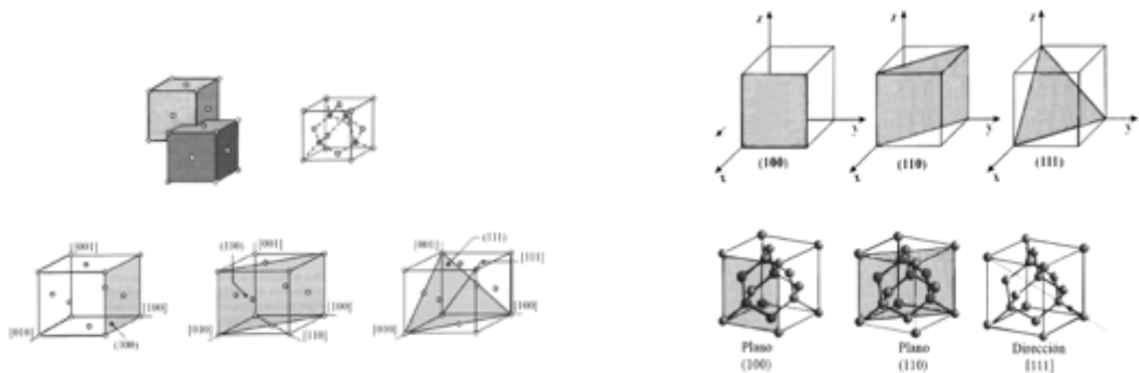
Estructura cristalográfica e índices de Miller para el silicio. El silicio representa una estructura tipo diamante con un parámetro de red a = 5.43 \text{ \AA} (Un Angstrom equivale a una diez millonésima parte de 1 mm)
